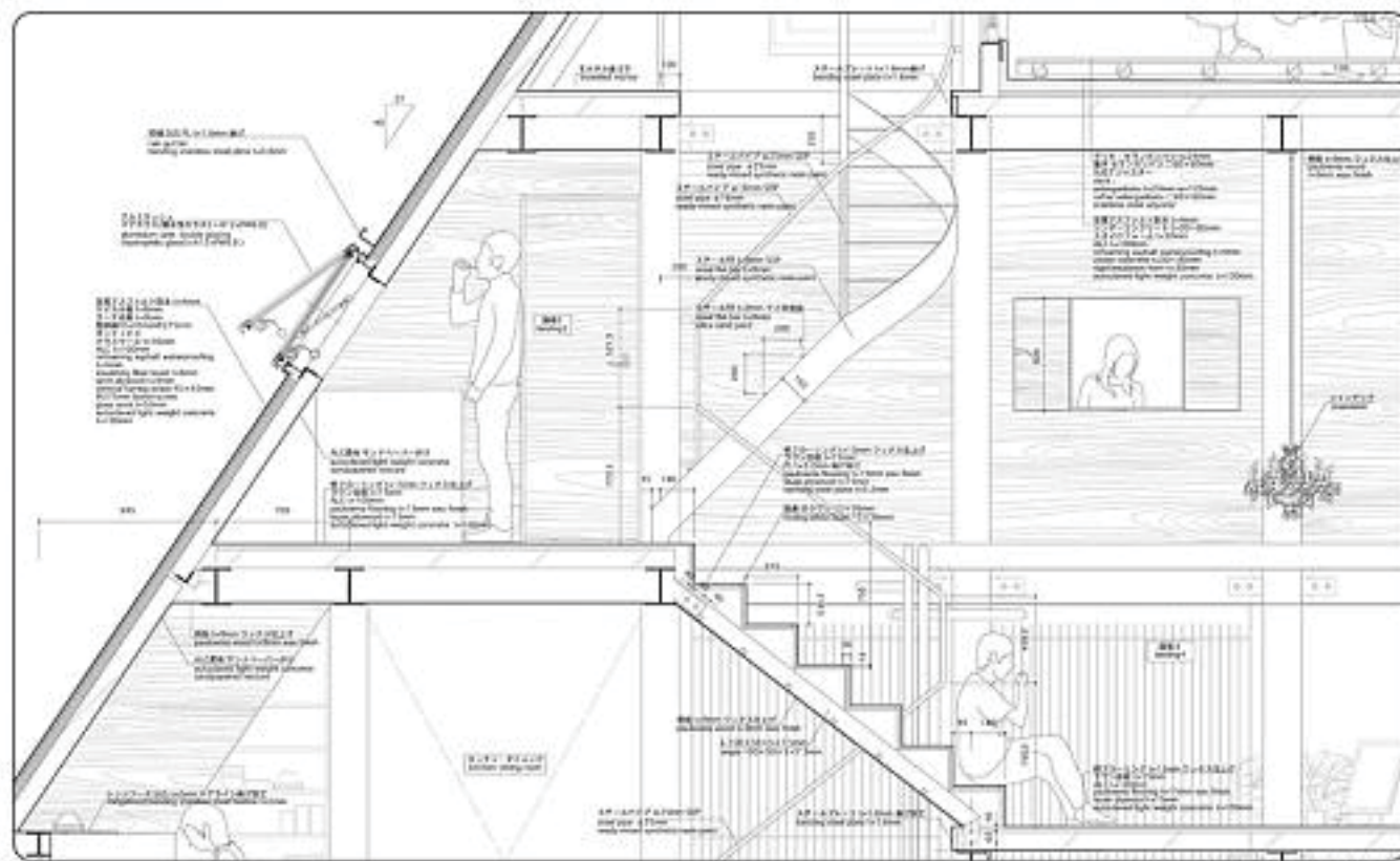
階段部 / 階段詳細図 / around stairs section detail 1:1/20
