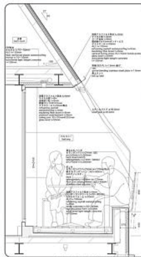
PLB-3-3 階段詳細図 / balcony section detail 1:1/20
