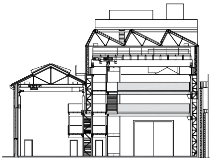
SEZIONE AA
